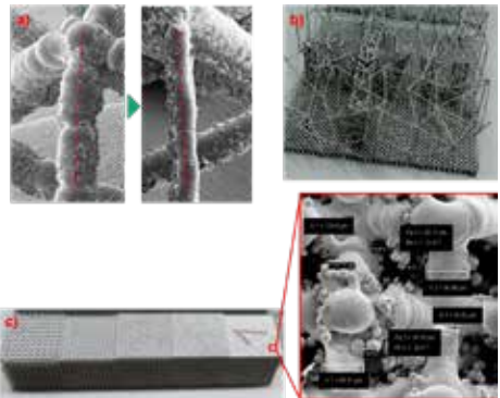
a) Qualitätsverbesserungen der Gitterstrukturen durch den angepassten Workflow. b) Demonstrator mit frei im Raum angeordneten Gitterstäben. c) filigranste auf konventioneller Anlagentechnik hergestellte Gitterstrukturen.
