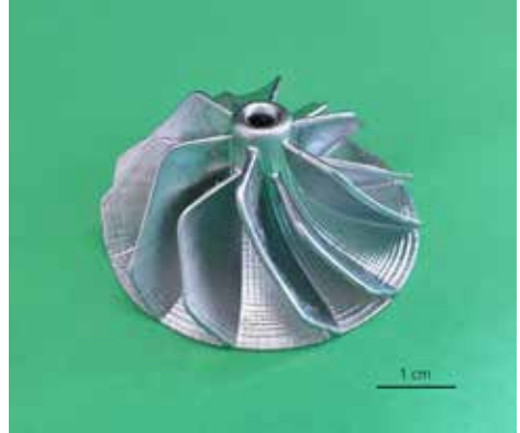
Propellerrad, hergestellt über AM-Formgebung und Gelcasting
