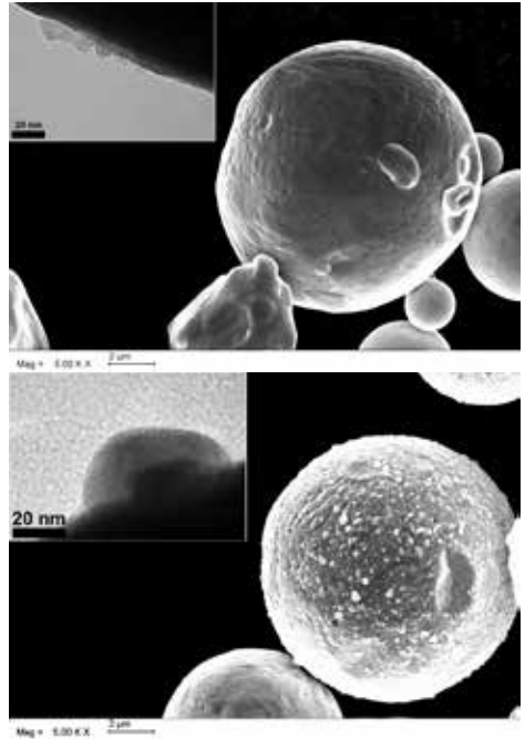
PVD-Beschichtung von Edelpulver (oben) – Einstellung der elektr. Leitfähigkeit durch eine Silberbeschichtung (unten)
