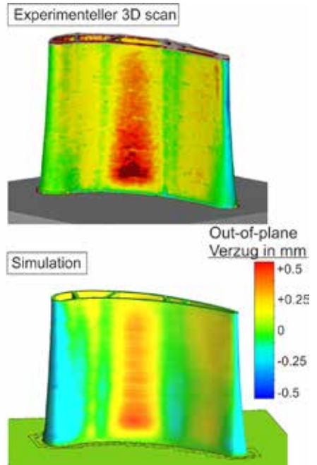
Der Vergleich von 3D-Scan und Simulation zeigt die gute Vorhersagequalität der Simulation.
