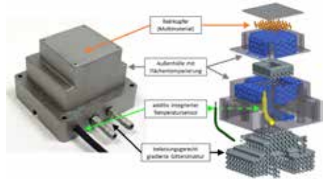
Funktionsintegriertes Spritzgießwerkzeug, Fertigteil (links) und Explosionsdarstellung (rechts)
