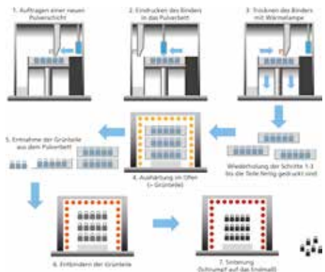
Schematische Darstellung der einzelnen Verfahrensschritte des Metal Binder Jettings
