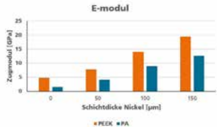
E-Modul von PEEK und Polyamid
