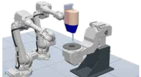
Kaltgasspritzen am Fraunhofer IGCV: Roboter mit Spritzpistole (mitte) vor dem Rotationstisch (rechts). Zweiter Roboter zum Integrieren von Komponenten oder anderen Funktionen (links)
