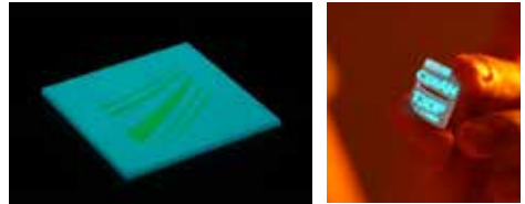
Additiv hergestellte, monolithische 2K-Sinterglasbauteile mit phosphoreszierender Komponente
